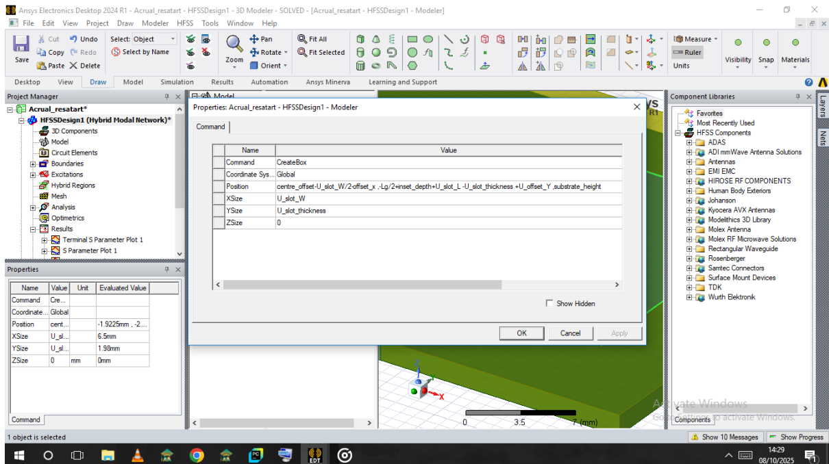
Figure 3.48: U-slot parameters
